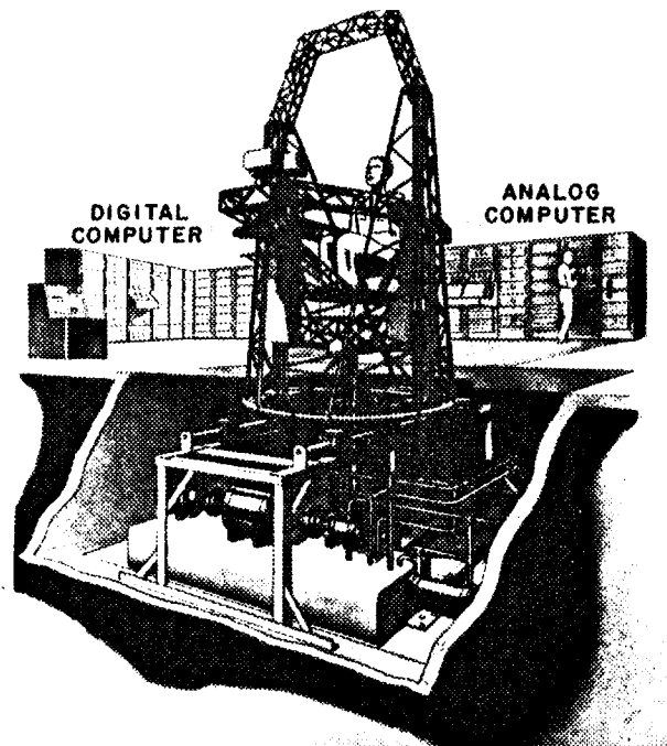
FIG. 15. SIMULATOR
