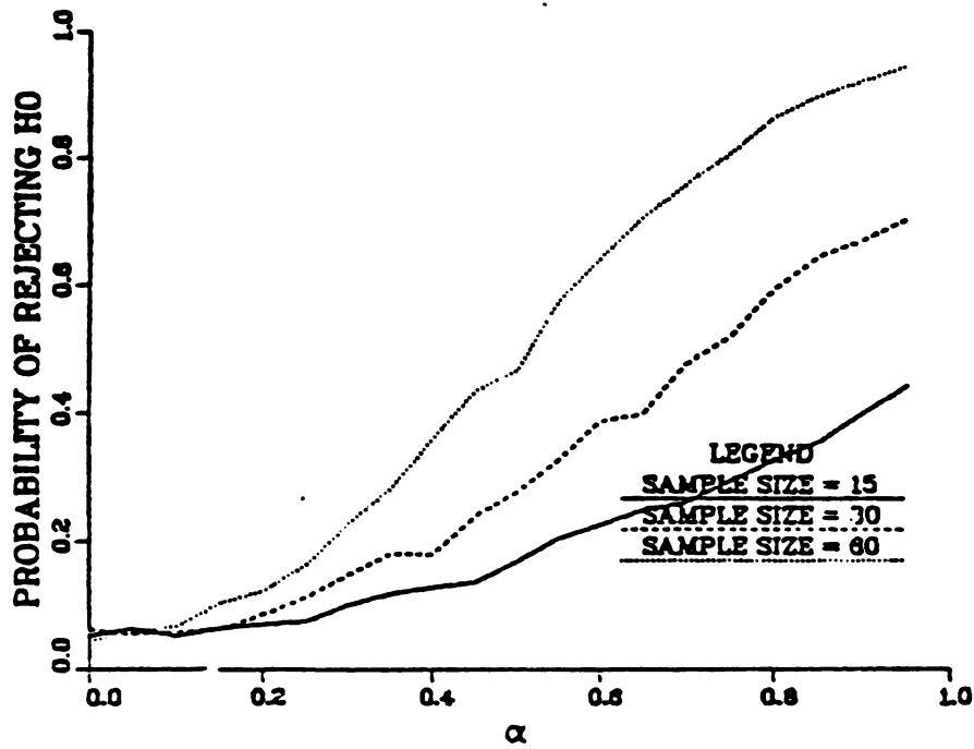
FIGURE 4: POWER OF 5%-LEVEL TEST H_0: F=G=CAUCHY(0,1) VS. H_1: F=CAUCHY(0,1), G=CAUCHY(\alpha \neq 0,1)
